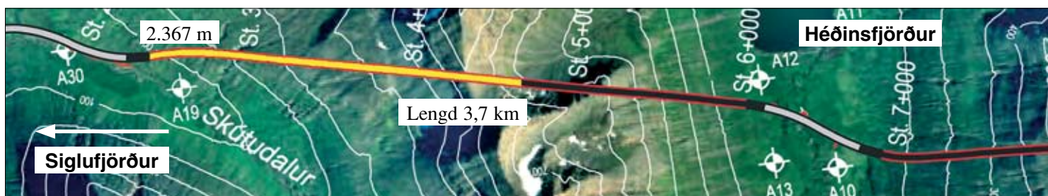
Staða framkvæmda við Héðinsfjarðargöng 10. sept. 2007. Búið er að sprengja 2.367 m í Siglufirði og 1.795 m í Ólafsfirði.
