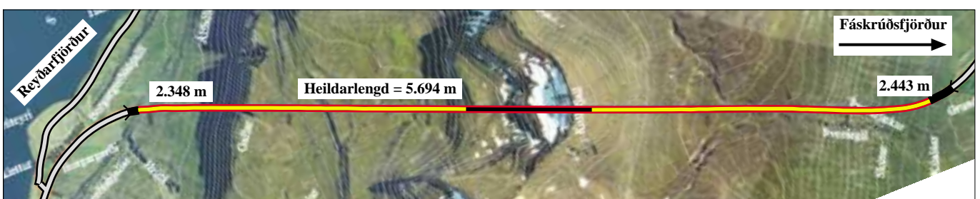
Staða framkvæmda við Fáskrúðsfjarðargöng 14. júní 2004. Samtals er búið að sprengja 4.791 m sem gerir 84,1%.
