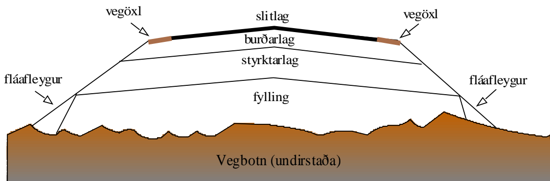
Mynd 5 Heiti hluta í veghloti (teikning ekki í réttum mælikvarða).
