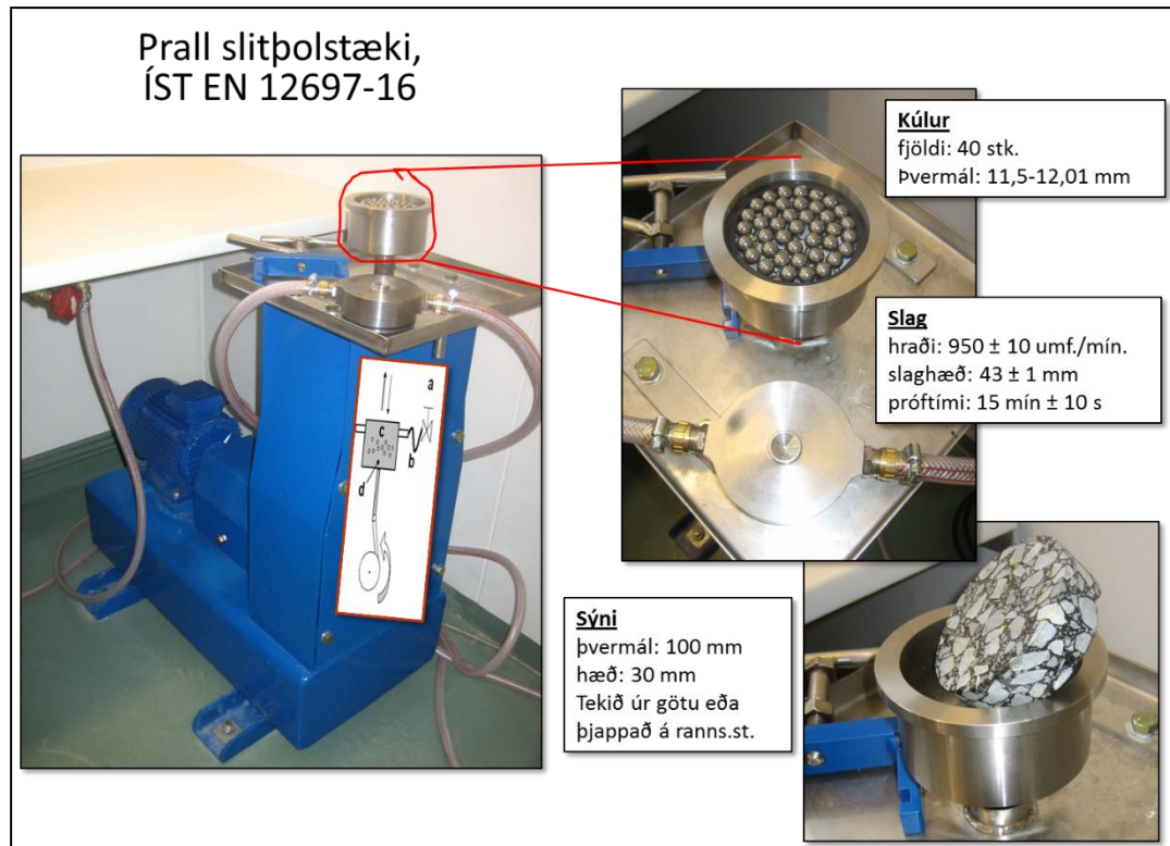
Mynd 79. Prall slitpolstæki og útskýringar á einstökum hlutum þess
