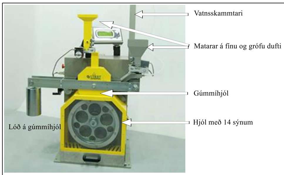
Mynd 50. Vélbúnaður til að slípa steinefnasýni
