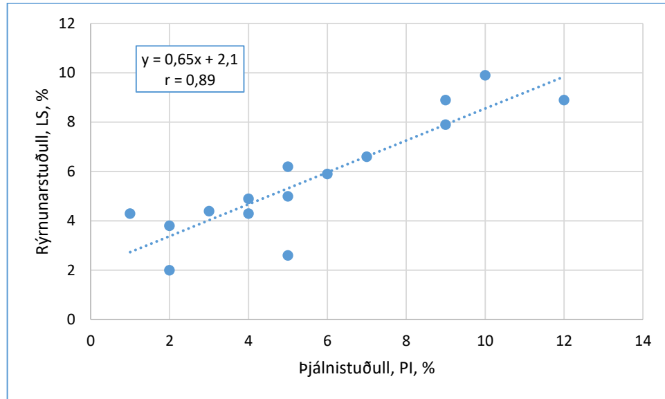
Mynd 23. Tengsl milli rýrnunarstuðuls og þjálnuðuðuls malarslitlagsefna
