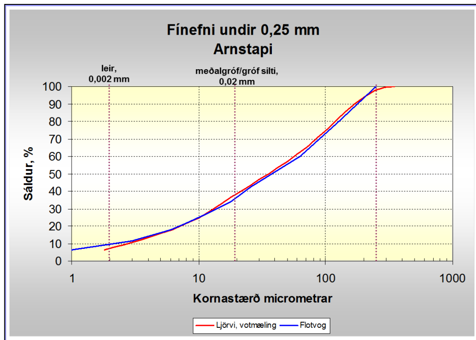
Mynd 7. Samanburður á kornastærðamælingu með flotvog (hydrometer) og ljörva (lasertæki)
