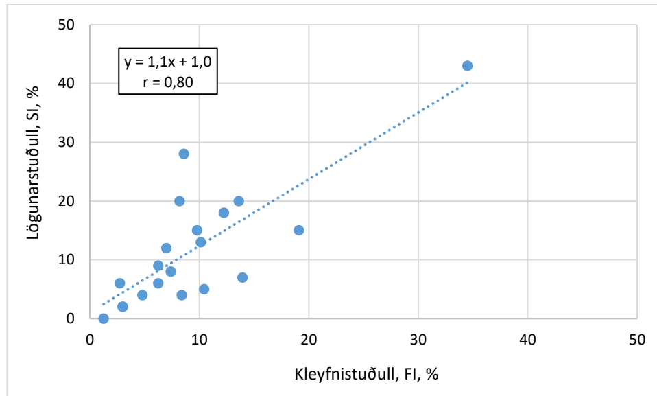
Mynd 30. Samband kleyfnistuðuls og lögunarstuðuls
