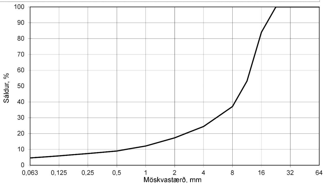
Mynd 4 a) Útskrift af niðurstöðum mælingar á kornadreifingu
