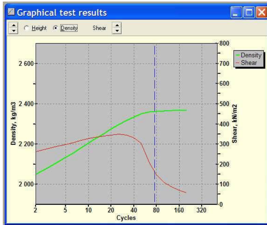
Mynd 77. Dæmi um útprentaðar niðurstöður úr prófun í Gyratory-þjöppu
