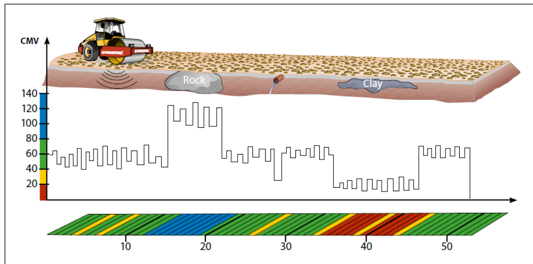
Mynd 64. Mótstöðukraftur jarðvegs mældur með þjöppumæli í valta
