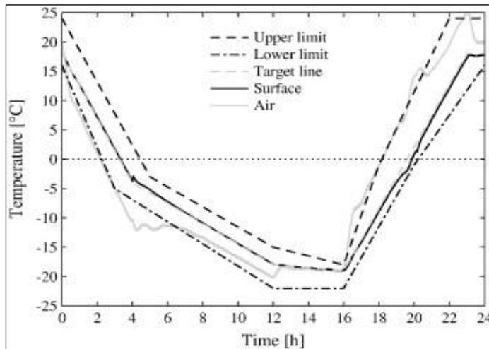
Mynd 84. Frostþolspróf (flögninarpróf) á steinsteypu, það sem flagnar við áraun er burstað frá
