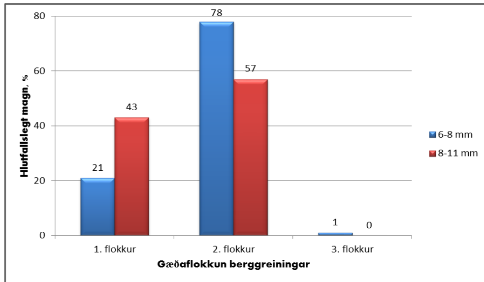
Mynd 28. Dæmi um tvær berggreiningar á sama sýni, en í mismunandi kornastærð
