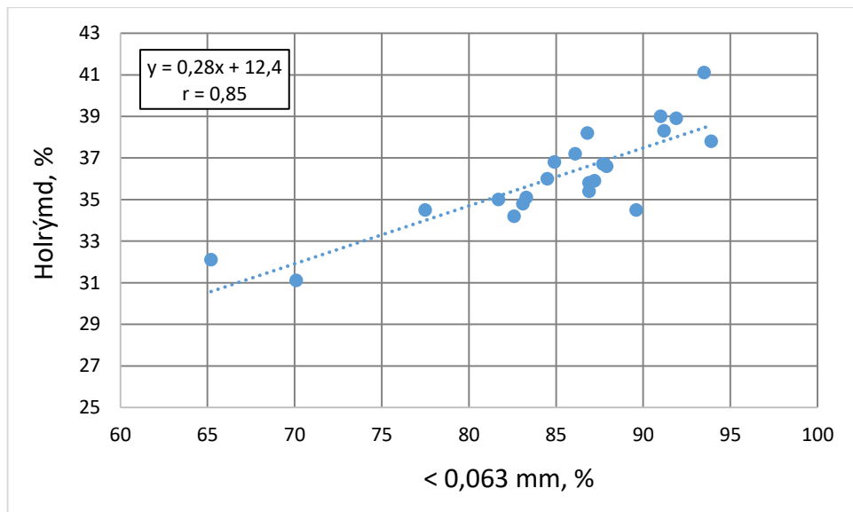
Mynd 18. Tengsl milli Rigden holrýmdar og efnis sem er < 0,063 mm
