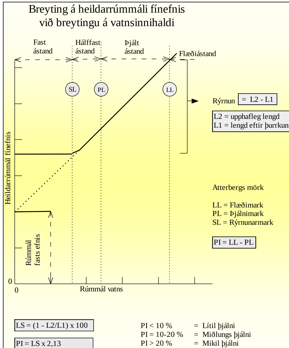
Mynd 19. Skilgreining Atterbergmarka
