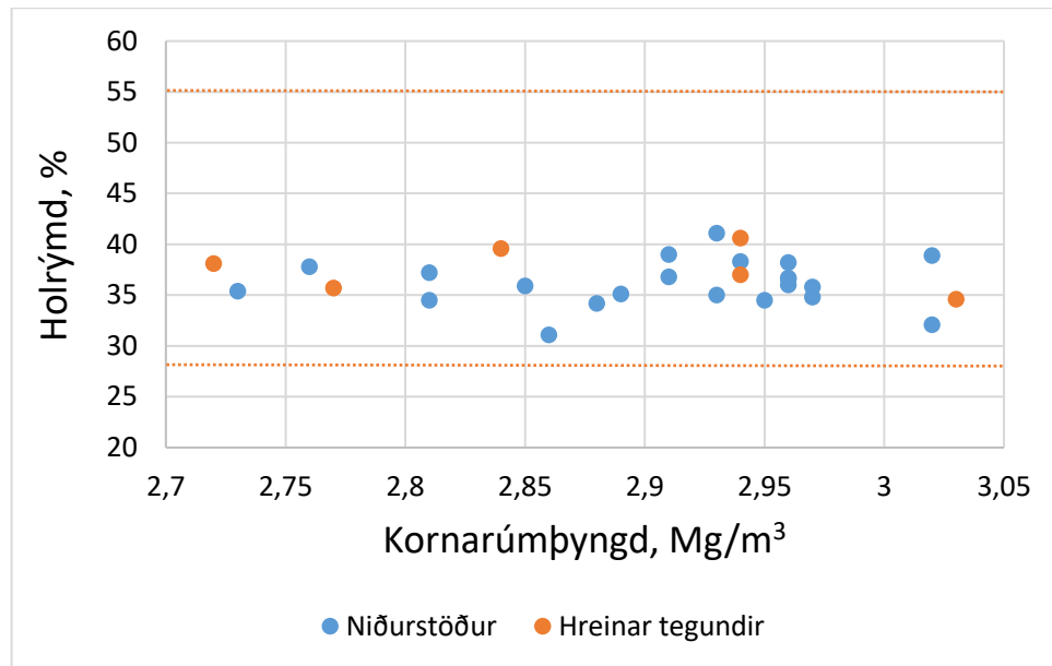
Mynd 16. Samanburður á holrýmd og rúmpýngd mélusýna
