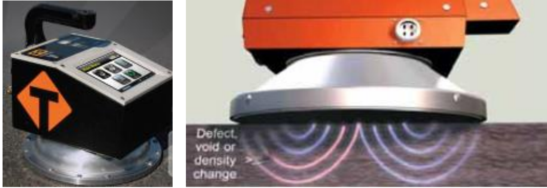
Mynd 67. Rafsegulmælir til mælingar á rúmþyngd/þjöppun
