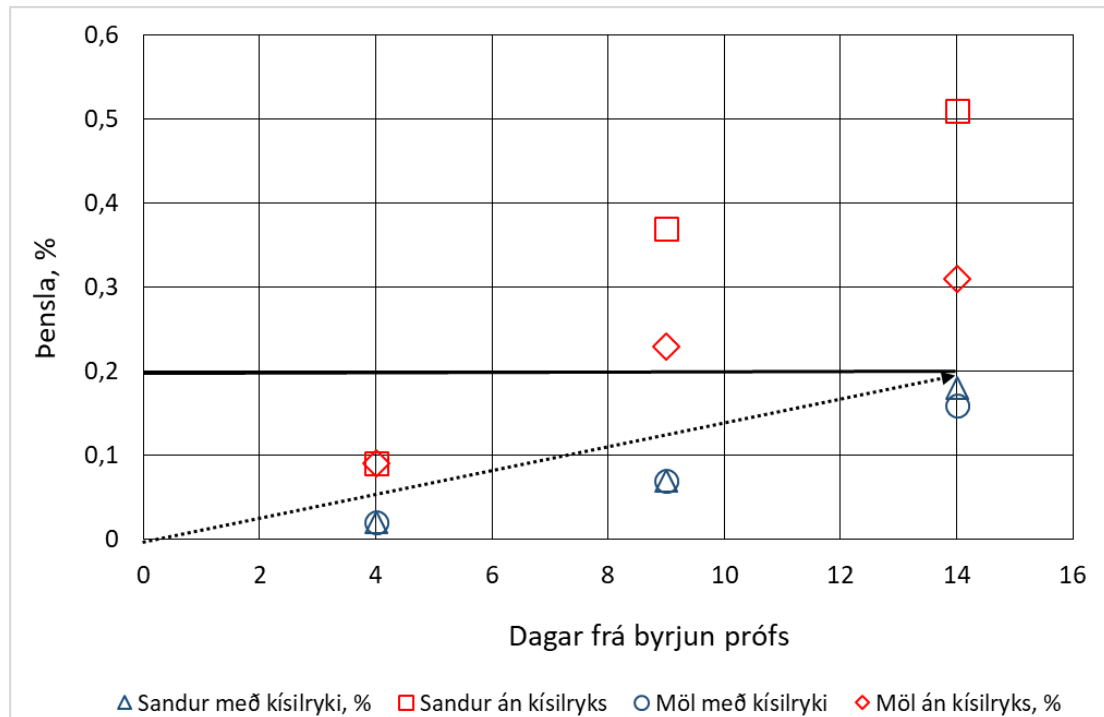
Mynd 53. Dæmi um hraðalkalípróf samkvæmt RILEM AAR-2 aðferðinni, með og án kísilyks (SF)
