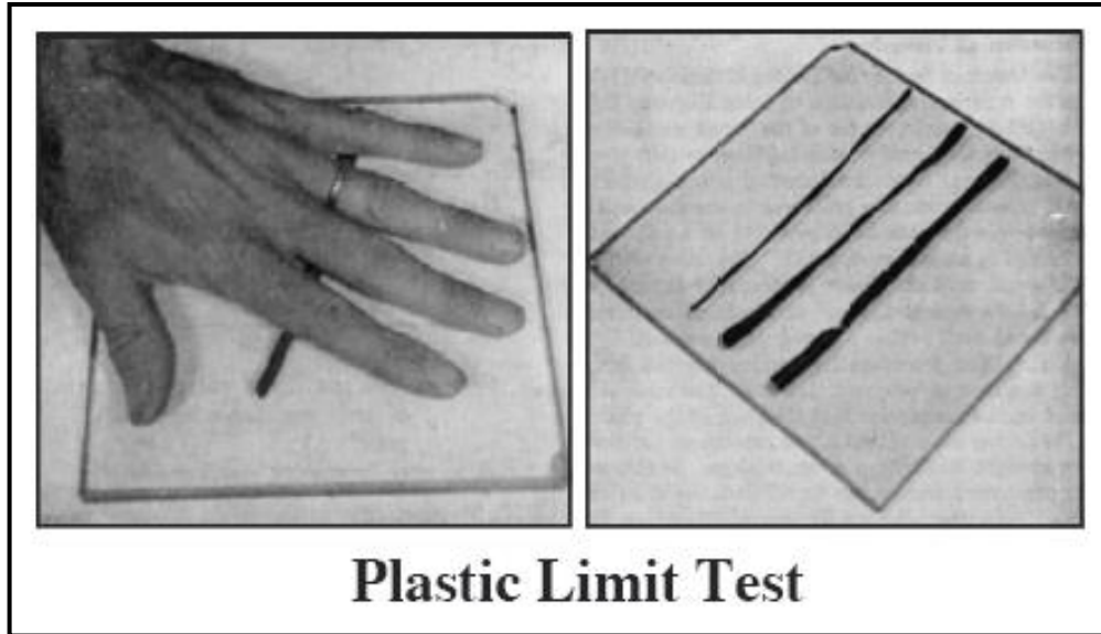
Mynd 21. Mæling á þjálnimarki
