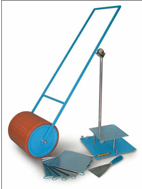
Mynd 48. Búnaður til að mæla viðloðun með Vialit plate-aðferðinni
