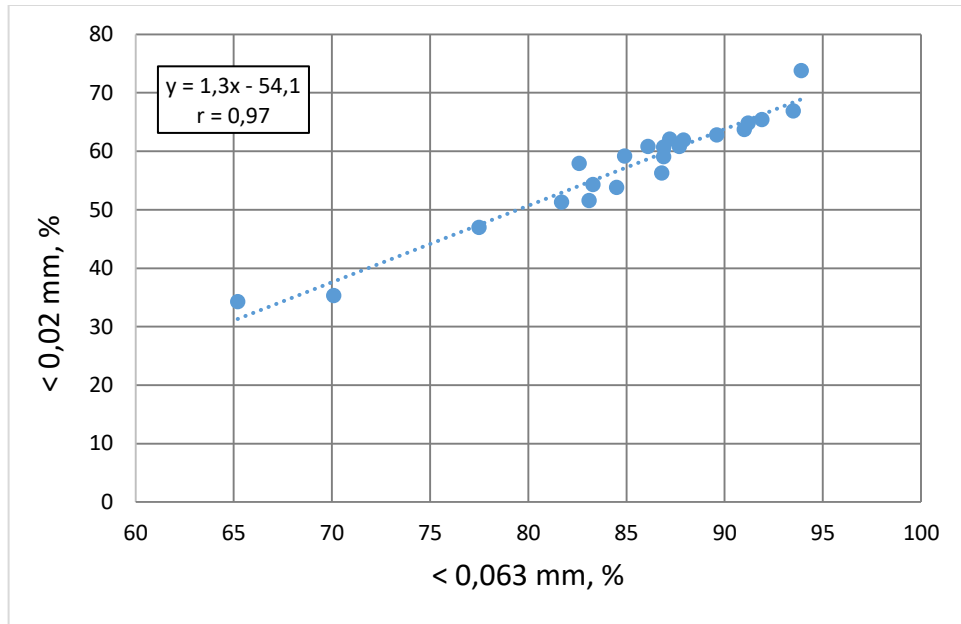
Mynd 17. Tengsl á milli magns <0,063 mm efnis og magns fínsýltis (<0,02 mm)
