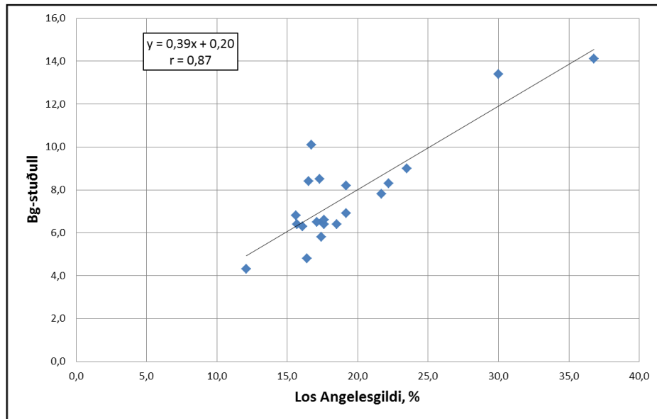
Mynd 37. Samband LA-gildis og Bg-stuðuls
