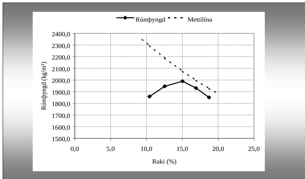
Mynd 58. Dæmi um samband rakainnihalds og þurrar rúmþyngdar
