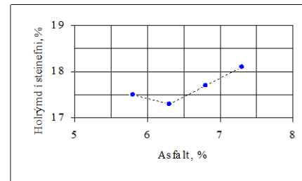
Mynd 73. Dæmi um niðurstöður Marshallprófs við hönnun malbiks
