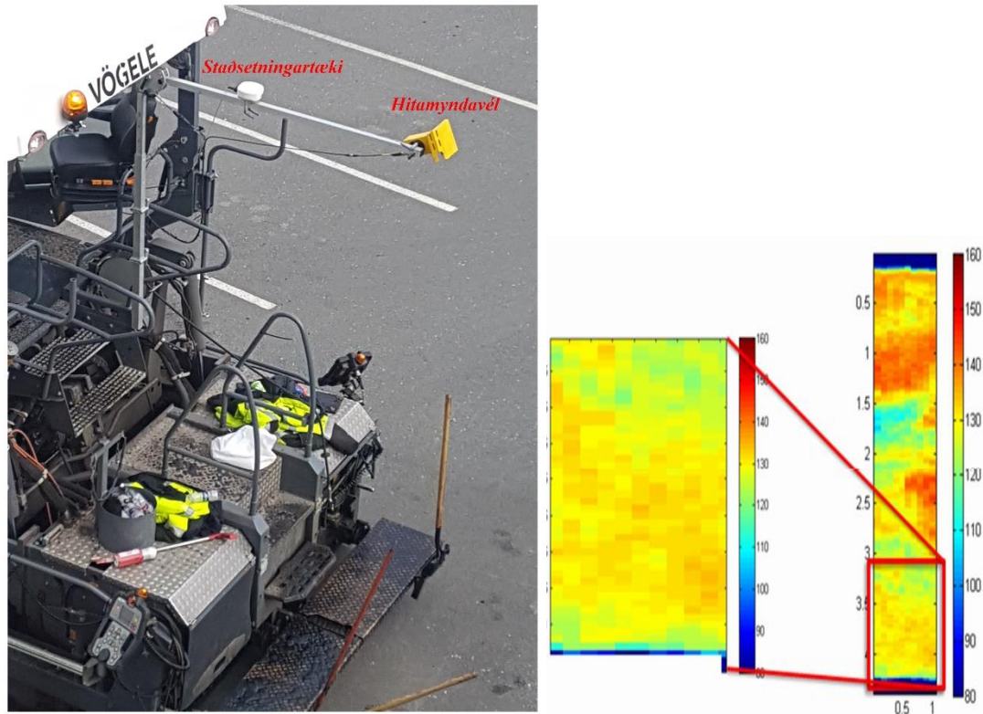
Mynd 81. Hitamyndavél og staðsetningartæki á útlagnarvél hérlandis og dæmi um útskrift
