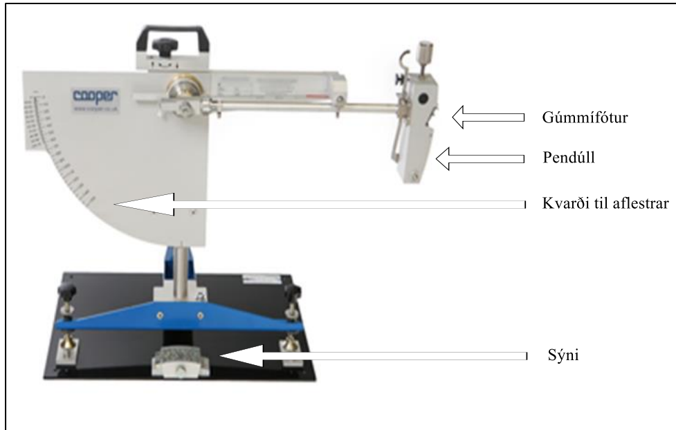
Mynd 51. Pendúll til að mæla hrjufleika steinefnasýna
