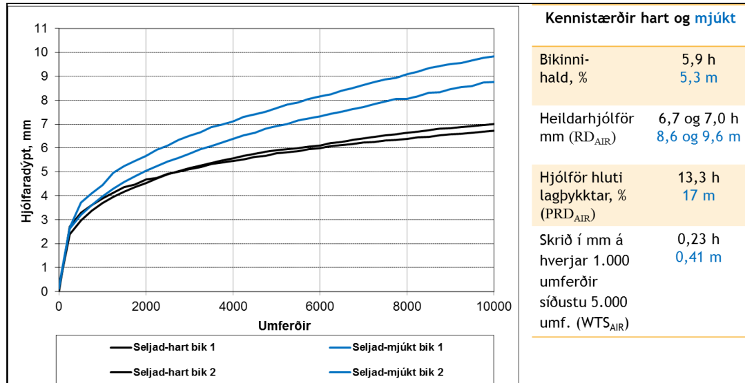
Mynd 70. Dæmi um framsetningu gagna úr hjólfaraþrófi
