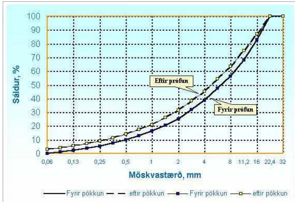
Mynd 341. Niðurstaða úr Bg prófi
