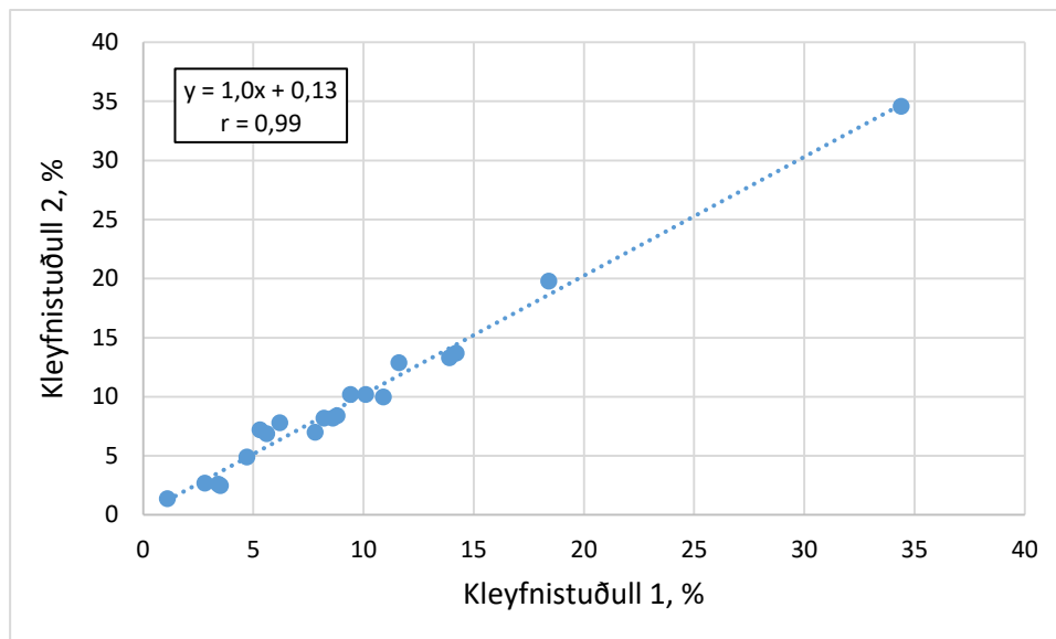
Mynd 33. Tengslin milli tveggja prófa með kleyfnistuðuls aðferðinni
