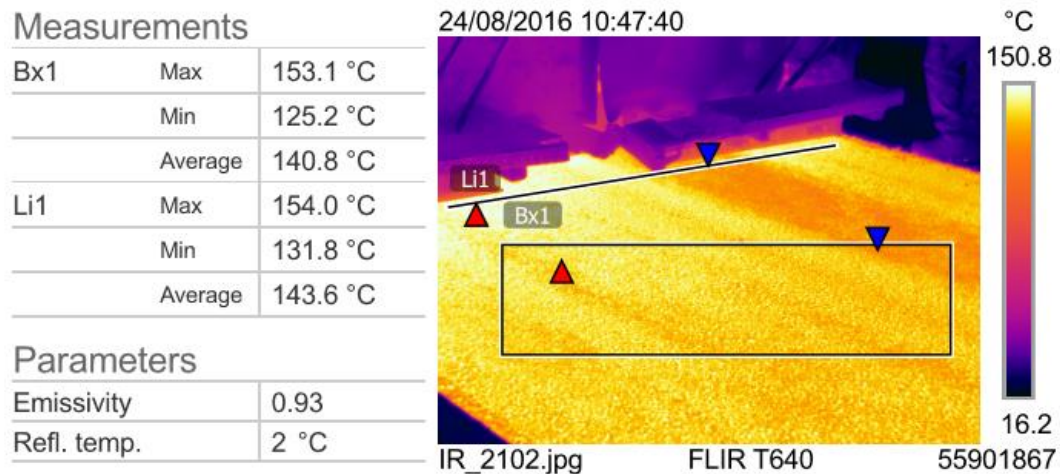
Mynd 80. Dæmi um hitadreifingu malbiks undan útlagnarvél
