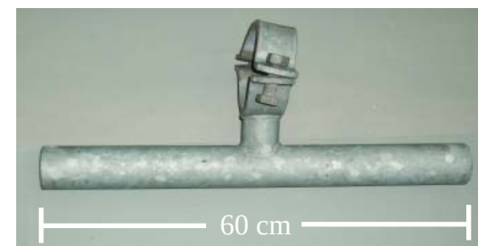
Einföld staurabaula með 75 mm röri
