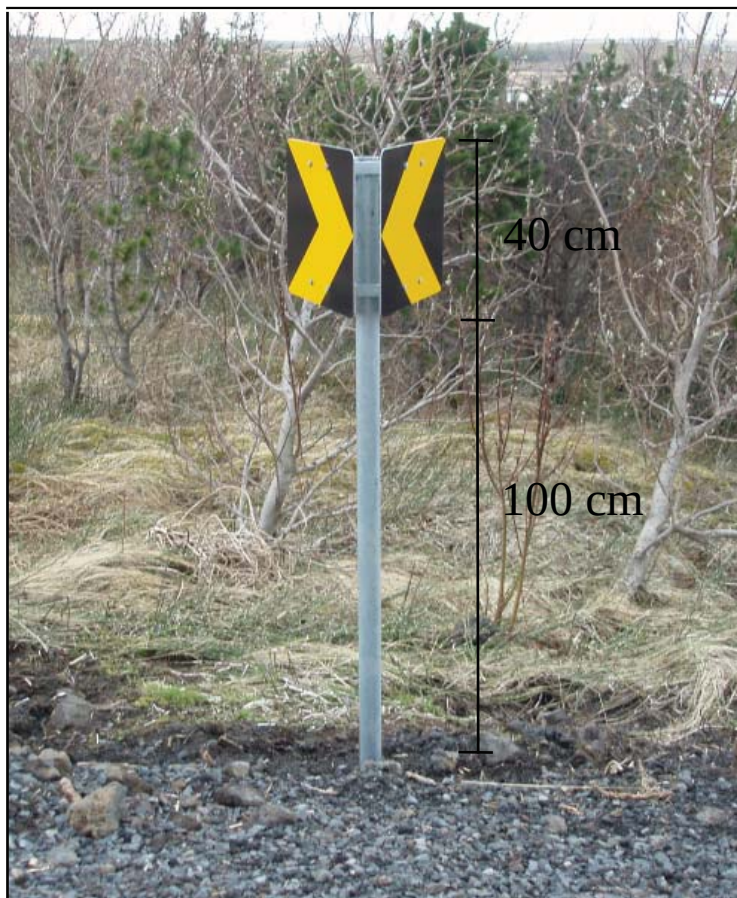
Uppsetning Stefnuörva
