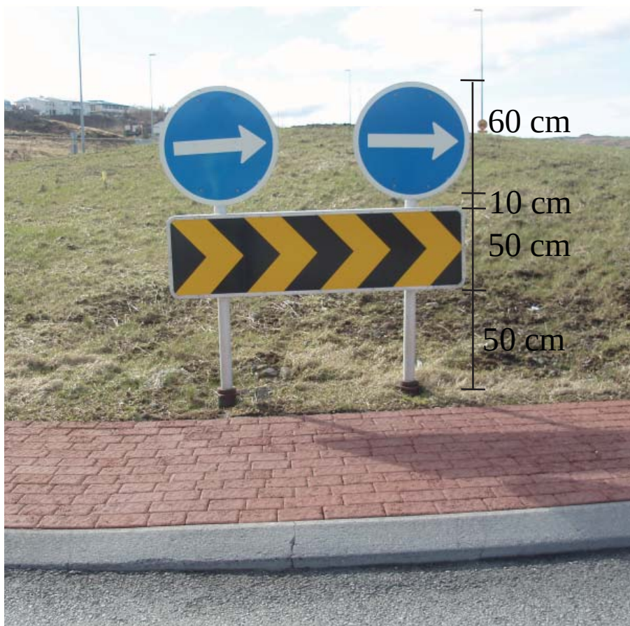
Uppsetning Þverslár
