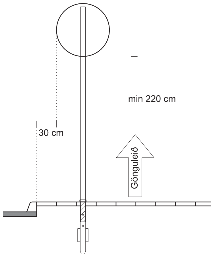
Uppsetning samsettra almenna umferðarmerkja
