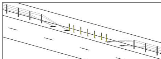
MYND 5-2 Útfærsla öryggis- og þjónustugáttar, op með plaststaurum sem hægt er að keyra niður.
