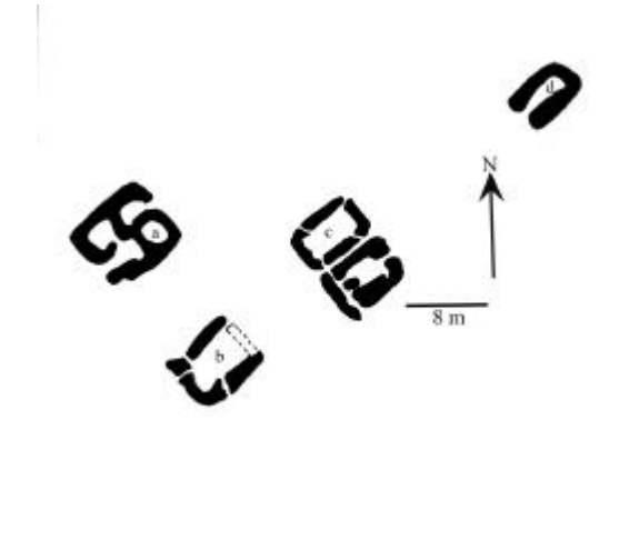
Péturssel. Teikning : Oddgeir Hansson.
