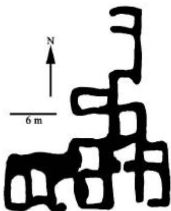
Krossavíkursel NÐ-078 :001. Teikning : Oddgeir Hansson
