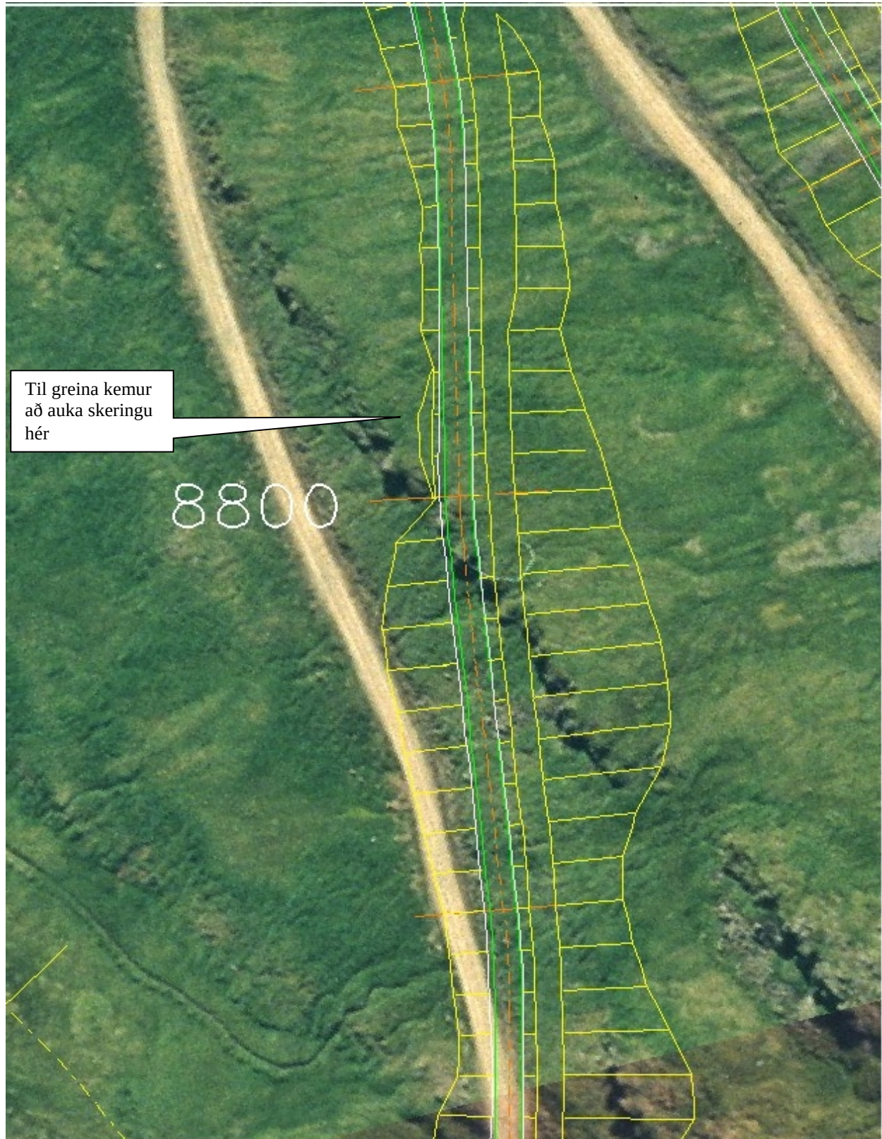
Bergskeringar milli stöðva 8600 og 8800 Í þessum kletturana er álitlegt berg í yfirbyggingu
