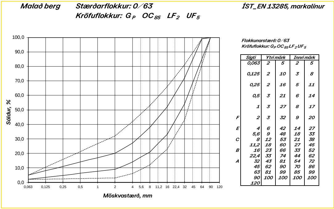
Mynd 5-14: Markalínur fyrir malað 63 mm berg og púkk í burðarlag
