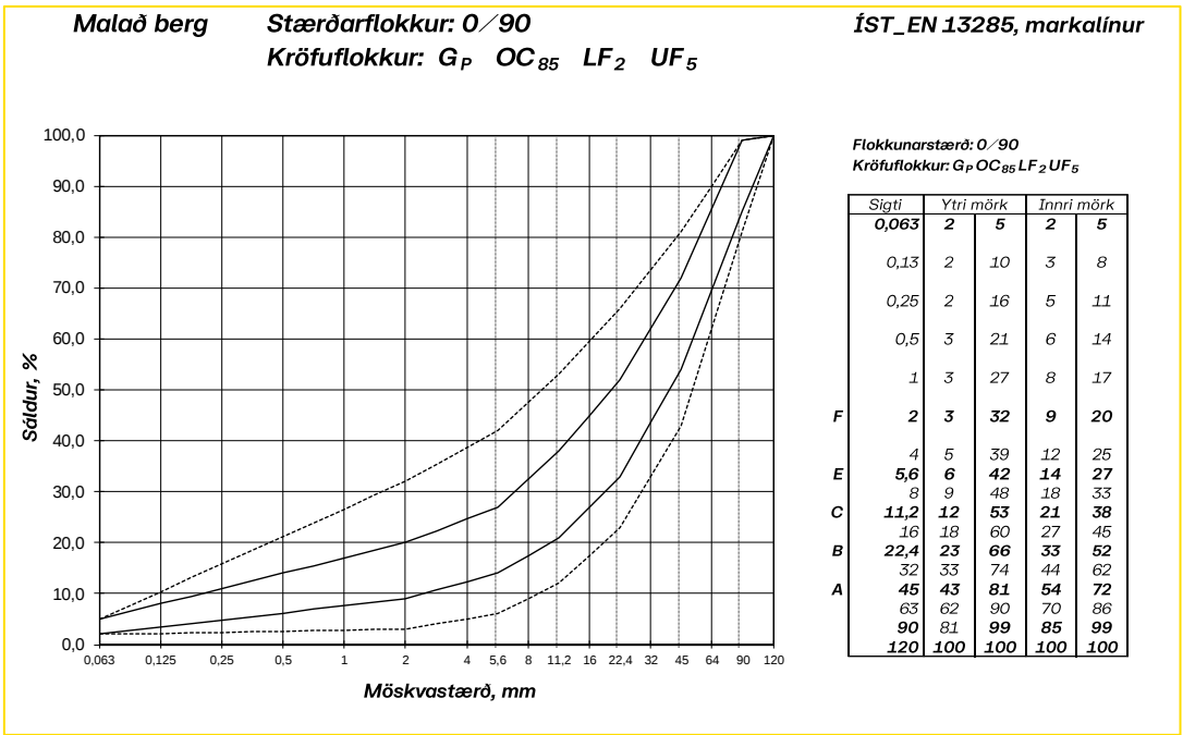
Mynd 5-15: Markalínur fyrir malað 90 mm berg og púkk í burðarlag
