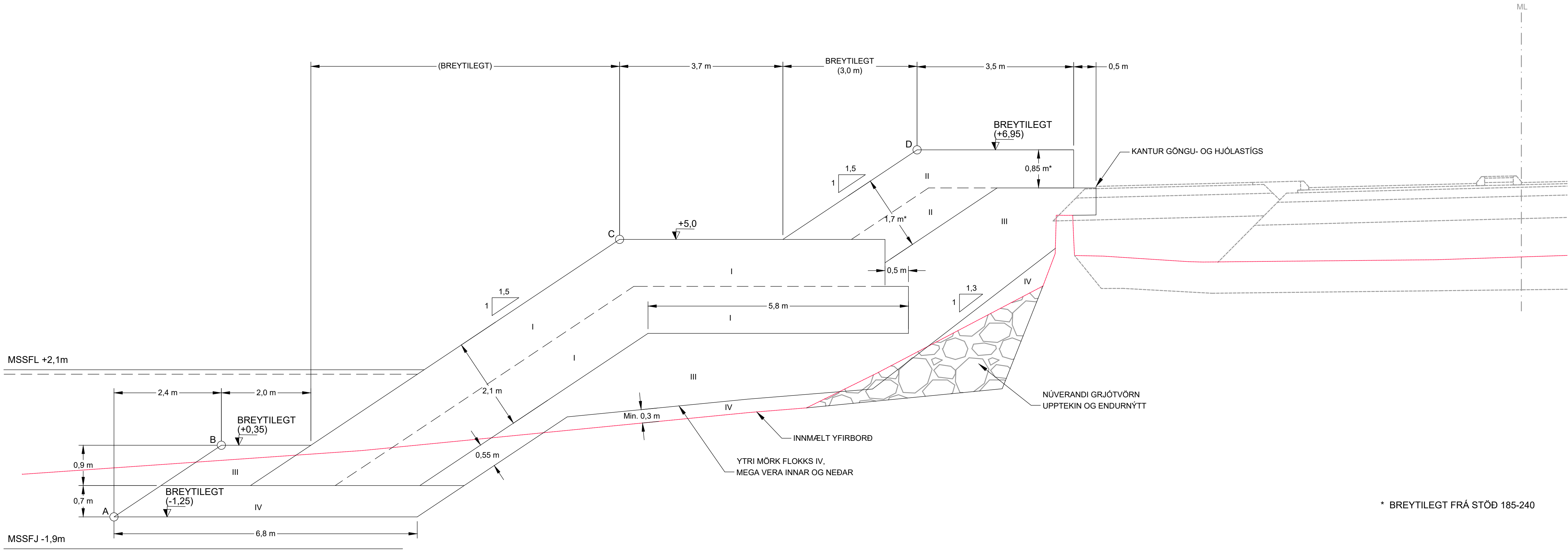
Kennisnið A, STÖÐ 185-470 (Teiknað í stöð 300)
