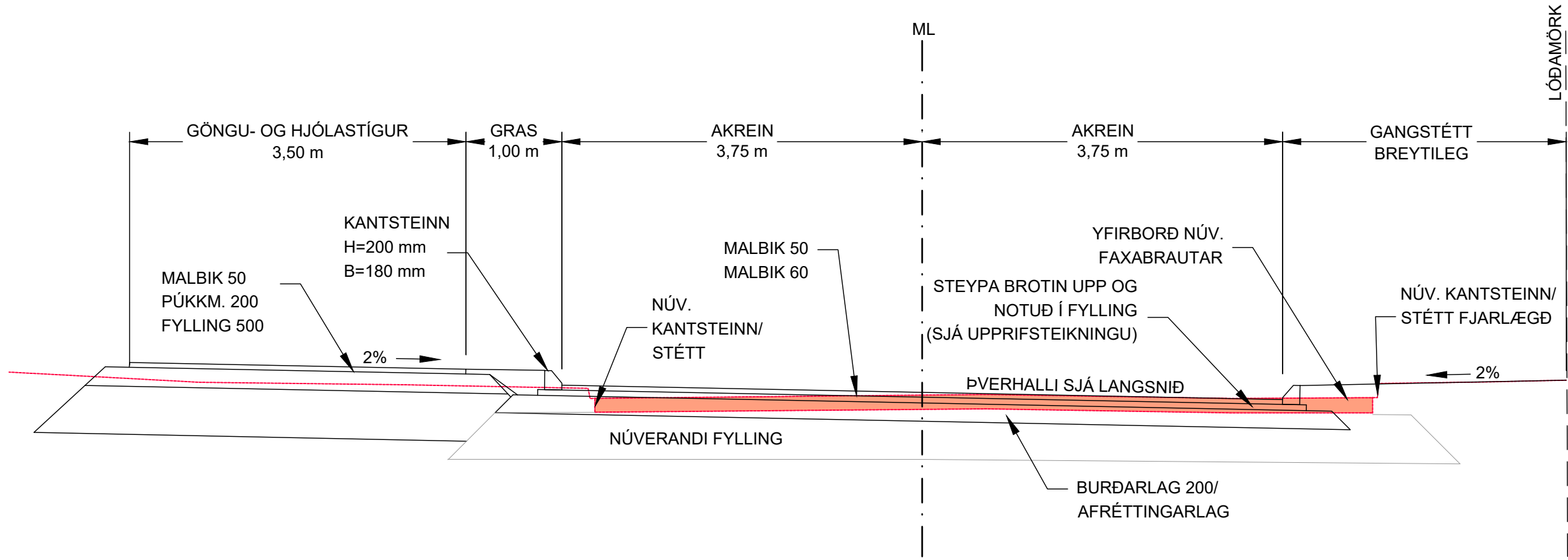
Kennisnið A, STÖÐ 30-140 1:50
