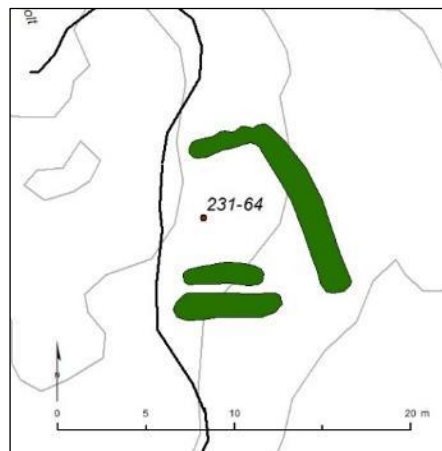
Mynd 28. Grjótagarður og garðlög (231-64), teiknað eftir uppmælingu.
