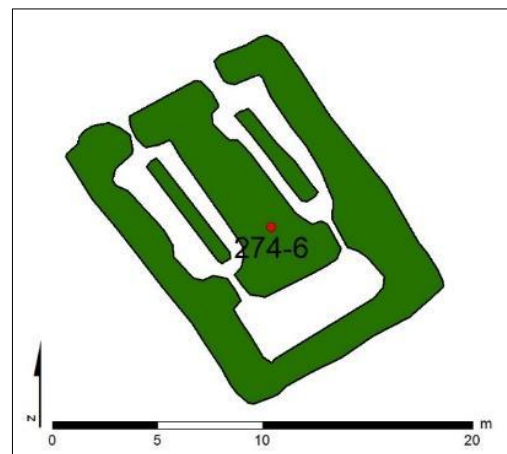
Mynd 190. Fjánhús og hlaða (274-6), teiknað eftir uppmælingu.
