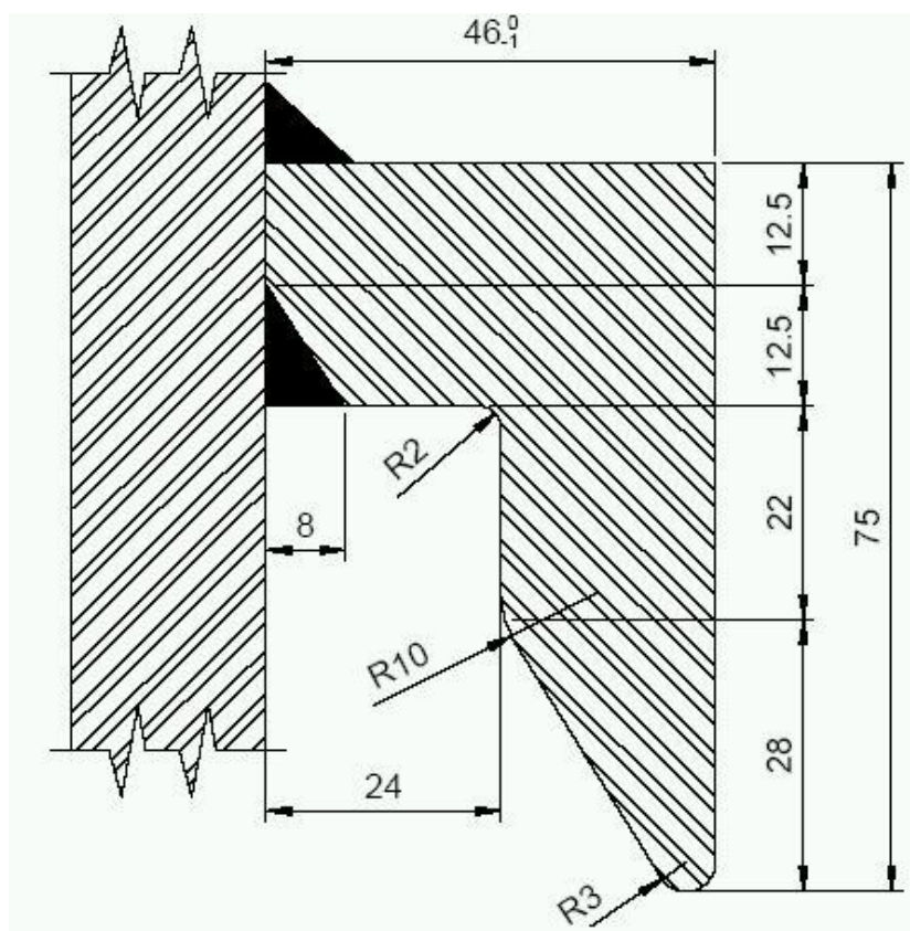
Mynd 2-6 Snið A-A (griphök).
