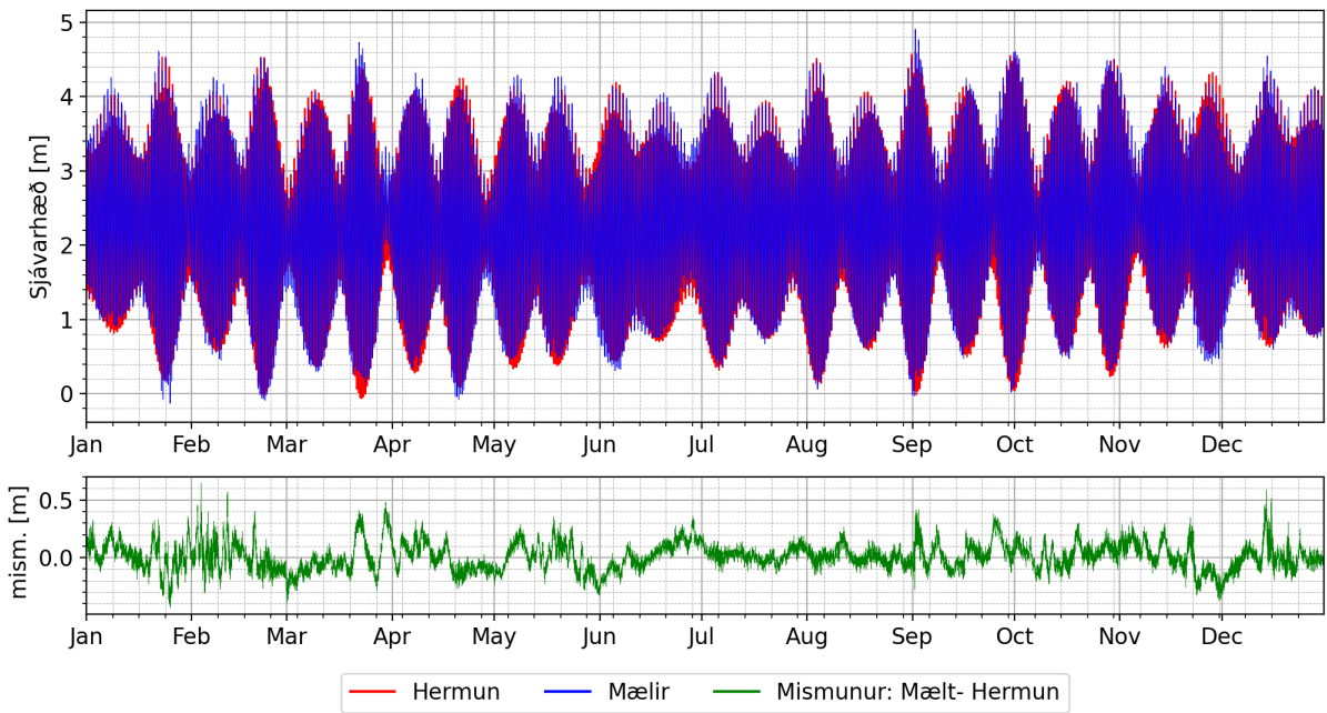
Sjávarhæðir Reykjavík - Miðbakki: 2023
