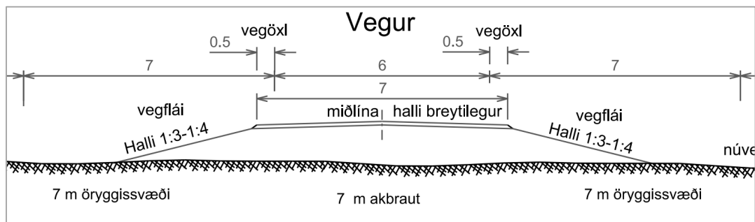
Mynd 18. Tengsl veggæðar, breiddar vegfláa og breiddar öryggissvæðis á 7 m vegi, vegtegund C 7 .
