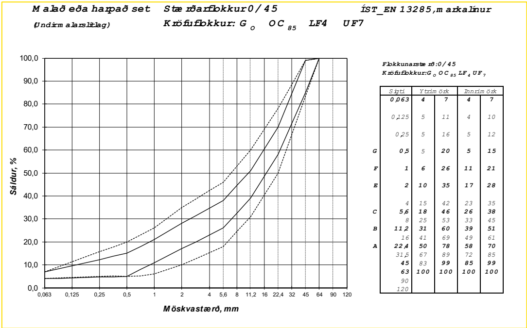
Mynd 5-17: Markalínur fyrir 45 mm malað eða harpað set í burðarlág malarvega
