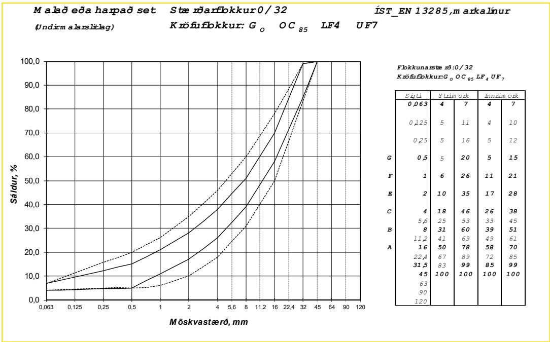
Mynd 5-16: Markalínur fyrir 32 mm malað eða harpað set í burðarlág malarvega
