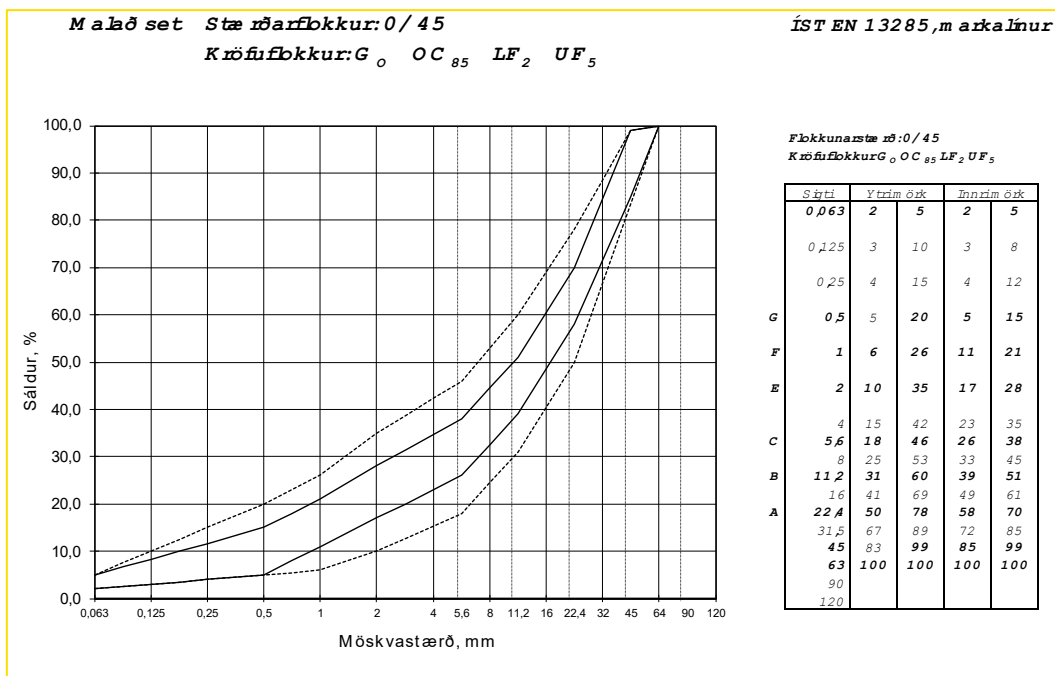
Mynd 5-9: Markalínur fyrir malað 45 mm set í burðarlag
