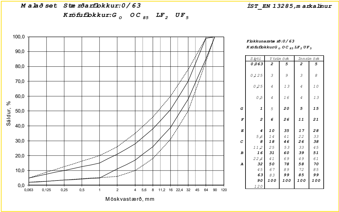
Mynd 5-10: Markalínur fyrir malað 63 mm set í burðarlag
