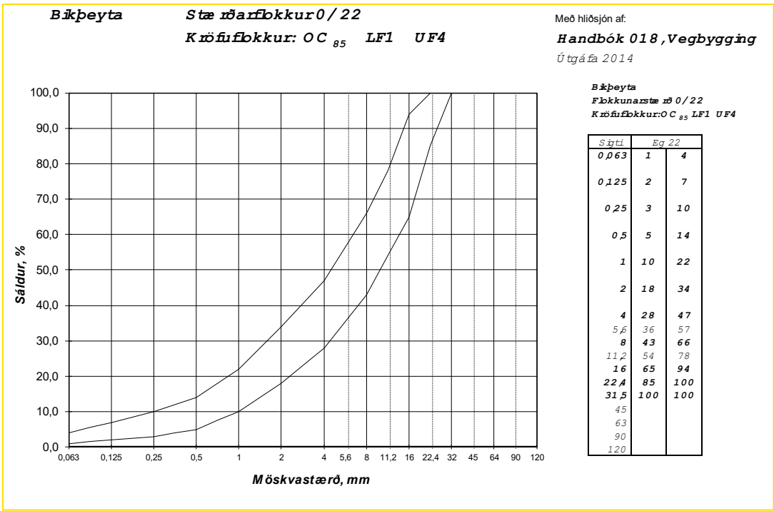
Mynd 5-22: Markalínur fyrir 22 mm steinefni (leiðbeinandi), fyrir bikpeytumalbik blandað í námu
