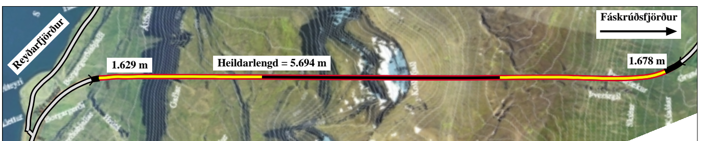
Staða framkvæmda við Fáskrúðsfjarðargöng 8. mars 2004. Samtals er búið að sprengja 3.307 m sem gerir 58%.
