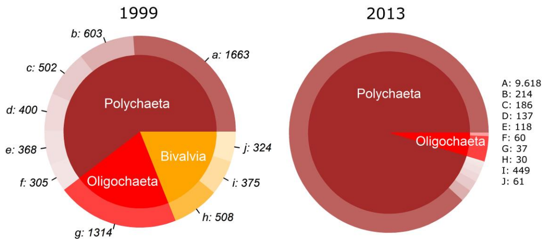
2. mynd. Tíu algengustu tegundir á botni Kolgrafafjarðar árin 1999 (Agnar Ingólfsson 1999) og 2013 (Valtýr Sigurðsson 2015) á þeim sjö stöðvum sem voru notaðar til samanburðar. Polychaeta=burstaormar, Oligochaeta=ánar, Bivalvia=samlökur. a: Polydora sp., b: Spionidae, c: Scalibregma inflatum, d: Chaetozone setosa, e: Levinsenia gracilis, f: Terebellides stroemi, g: Oligochaeta, h: Nuculana tenuis, i: Mytilus edulis, j: Macoma calcaria. A: Capitella capitata, B: Spionidae, C: Chaetozone setosa, D: Harmothoe sp., E: Microphthalmus aberrans, F: Eteone longa, G: Mediomastus fragilis, H: Aricidea suecica, I: Oligochaeta, J: Tubificoides kozloffii. Tölurnar standa fyrir fjölda dýra á fermetra. Heiti dýra sem voru á meðal 10 algengustu bæði árin eru lituð blá.
