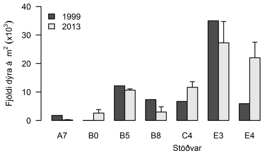
4. mynd. Þéttleiki einstaklinga (fjöldi á fermetra) á botni Kolgrafafjarðar árin 1999 og 2013. Yfirgnæfandi meirihluti dýra í sýnunum árið 2013 voru af aðeins einni tegund, burstaorminum Capitella capitata .
