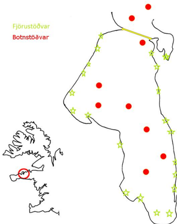
1. mynd. Botnsýni voru tekin á 7 stöðvum sunnan vegfyllingar og brúar í Kolgrafafirði og tveim stöðvum utan brúar (rauðir punktar). Fjörusýni voru tekin á 21 stöð vítt og breitt um fjörðinn (grænar stjörnur).
