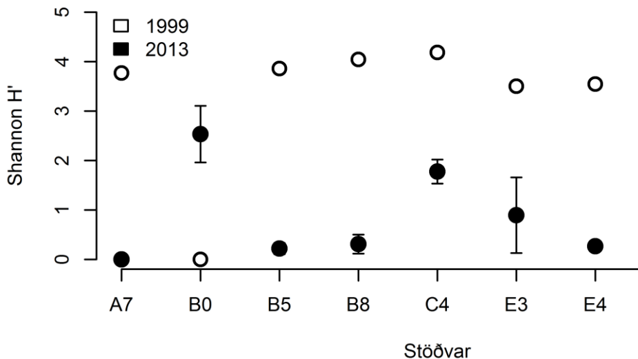
3. mynd. Líffræðileg fjölbreytni (Shannon H' ), reiknuð fyrir sýnatökustöðvarnar árin 1999 og 2013. Fjölbreytileiki dýra minnkaði verulega eftir síldardauðann.
