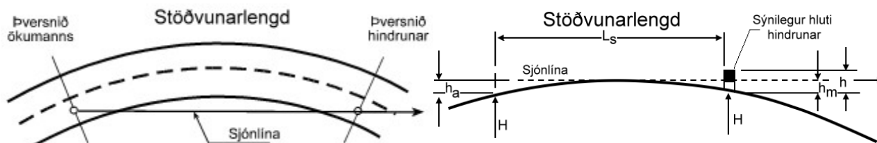
Mynd 3.6.2-1 Stöðvunarlengd í láréttum og lóðréttum fleti
