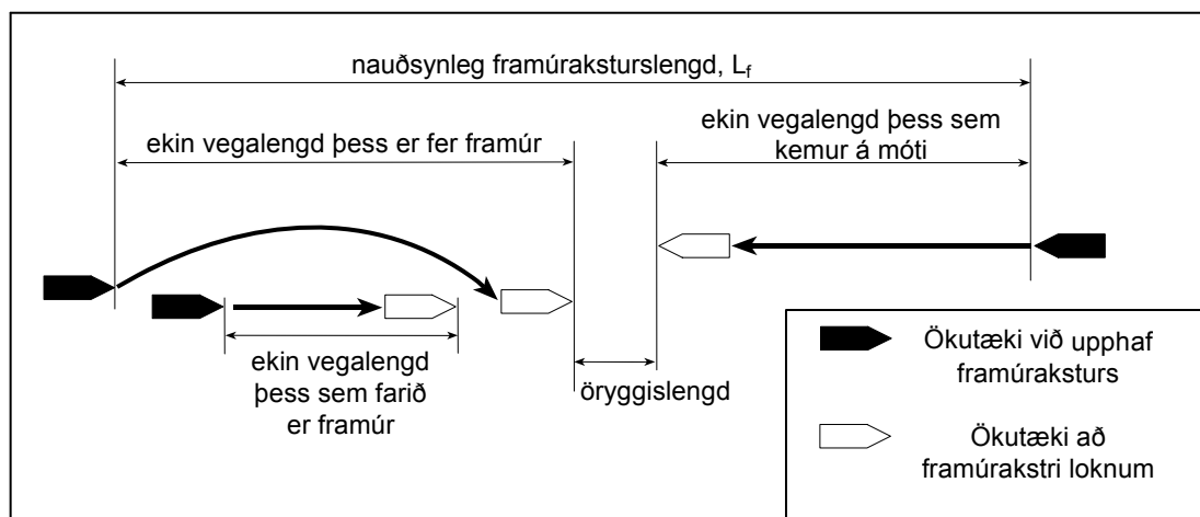
Mynd 3.6.4-2 Nauðsynleg framúraksturslengd, L_f
