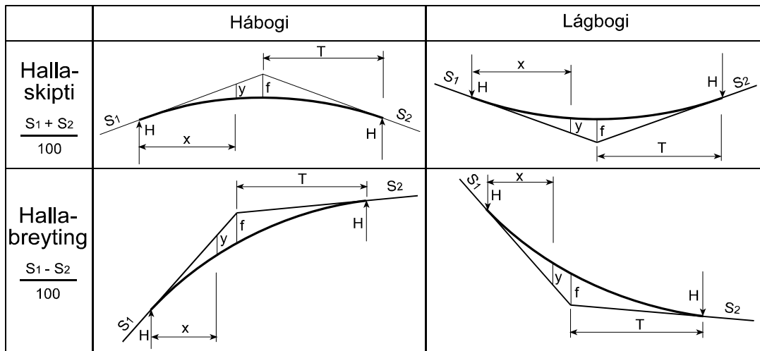
Mynd 3.4.2-1 Skýringar á stærðum í há- og lágboga, S er langhalli, T er snertill og H er radius
