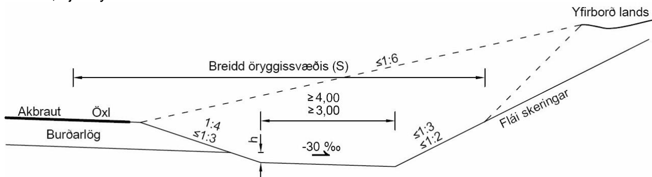
Mynd 2.4.3-1 Skering í lausan jarðveg
