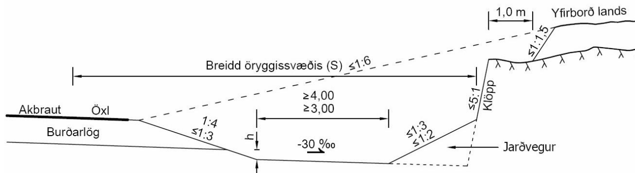
Mynd 2.4.3-2 Skering í berg
