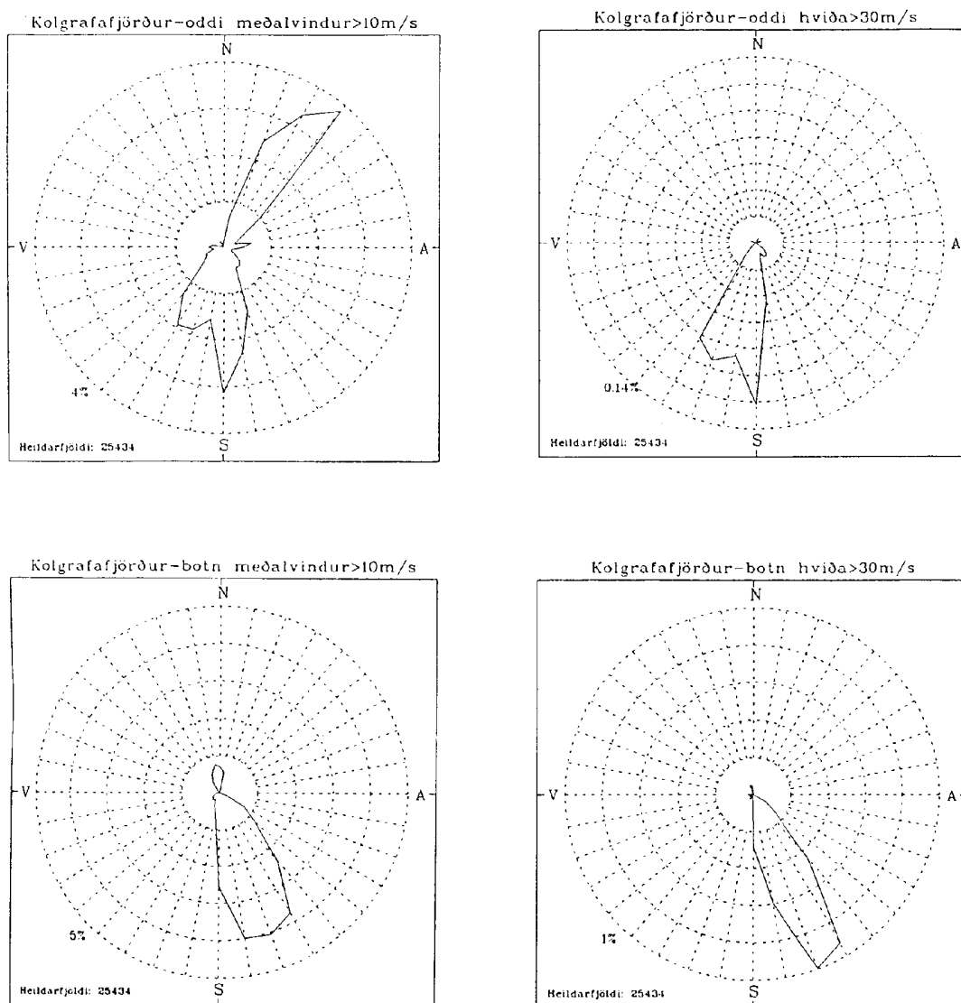
Mynd 26. Vindrósir sem sýna tíðni vindáttar er meðalvindur er yfir 10 m/s annars vegar og hins vegar ef hviður eru yfir 30 m/s á stöðvunum tveimur í Kolgrafafirði.
