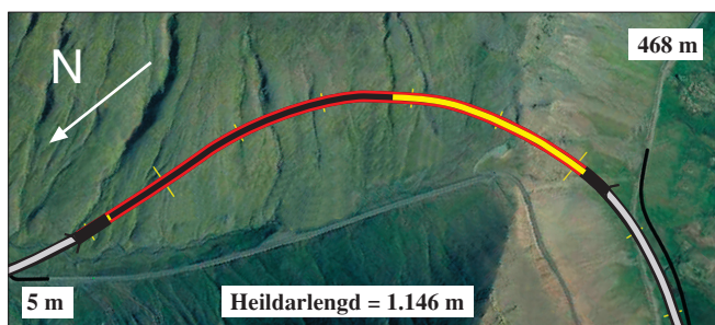
Staða framkvæmda við Almannaskarðsgöng 10. ágúst 2004. Samtals er búið að sprengja 473 m sem gerir 41%.
