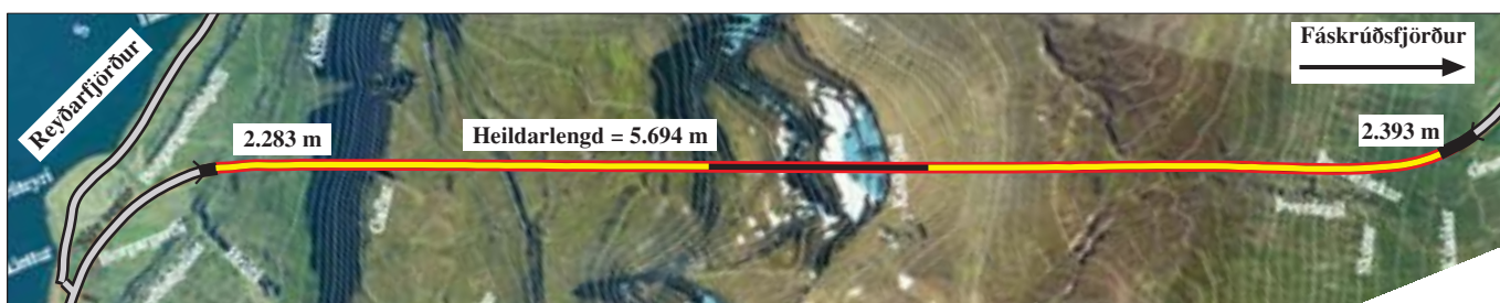
Staða framkvæmda við Fáskrúðsfjarðargöng 7. júní 2004. Samtals er búið að sprengja 4.676 m sem gerir 82,1%.
