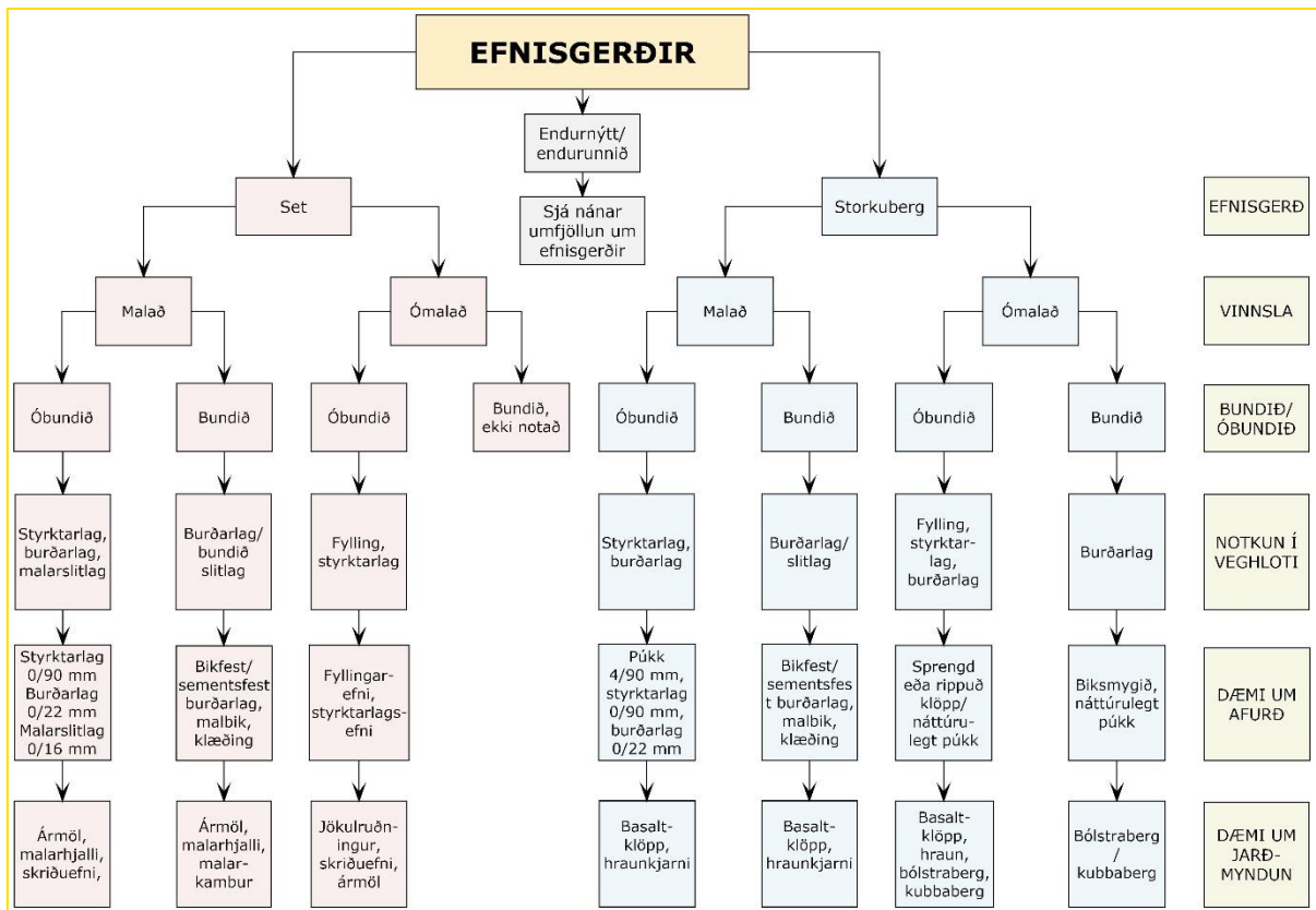
Mynd 1 Efnisgerðir í vega- og gatnagerð
