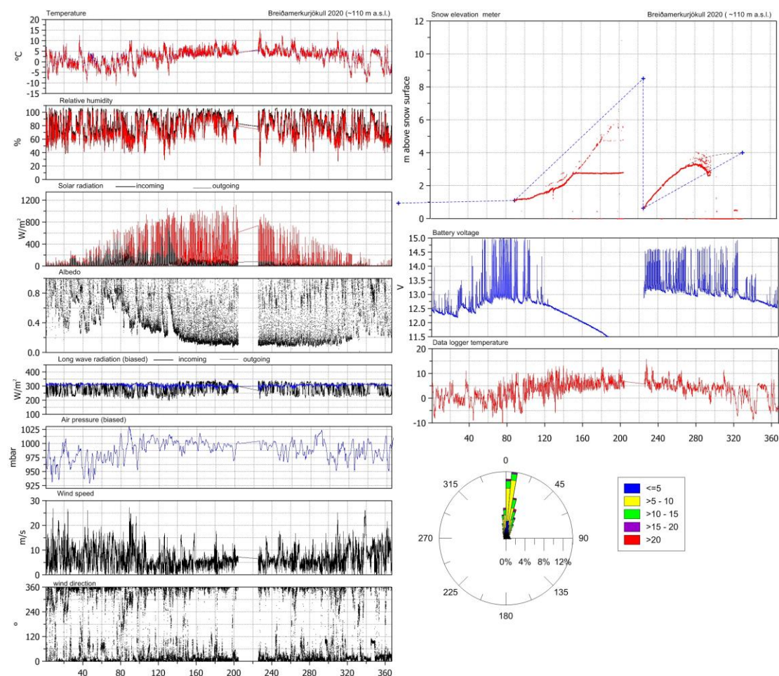
13. mynd. Mældir veðurþættir á veðurstöð í um 110 m hæð á sporði Breiðamerkurjökuls.
