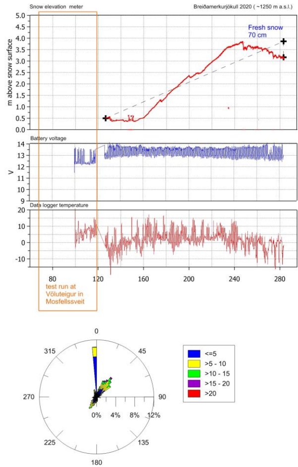
14. mynd. Mældir veðurþættir á veðurstöð í um 1250 m hæð á austurstraumi Breiðamerkurjökuls.
