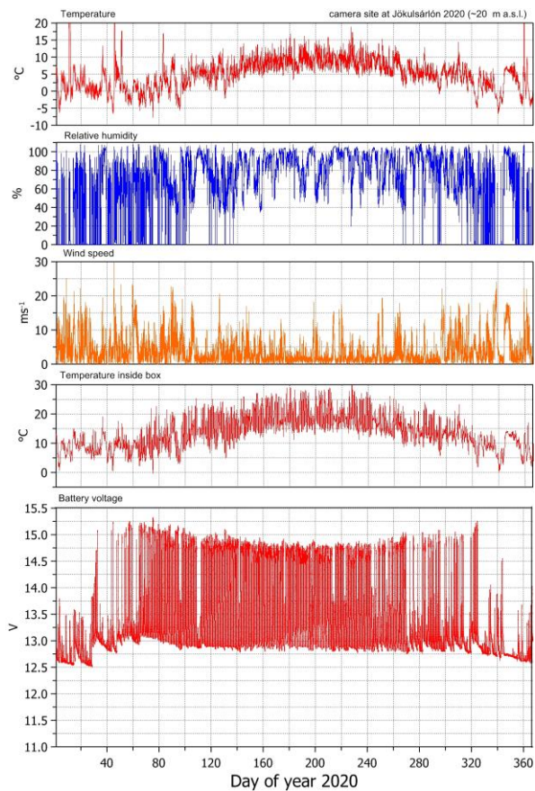
15. mynd. Lofthiti, raki og vindstyrkur mælt á veðurstöð í um 20 m hæð við NA jaðar Jökulsárlóns.
