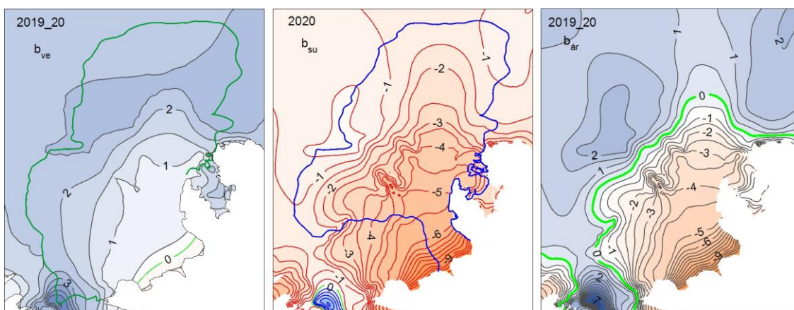
3. mynd. Dreifing vetrar- (vinstri) sumar- (miðja) og ársafkomu (hægri) á Breiðamerkurjökli 2019-20 (afkoma í m vatns). Ísasvið Breiðamerkurjökuls er sýnt með grænni línu (vinstri ramma) og vatnasvið Jökulsárlóns á Breiðamerkursandi með blárrí línu (miðju ramma).
