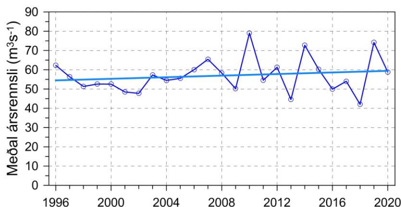
7. mynd. Meðalársafrennsli (á jökulári þ.e. október til september) yfirborðsleysingarvatns (metið úfrá sumarafkomu) til Jökulsárlóns sumurin 1996 til 2020.
