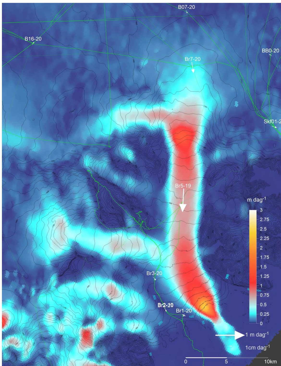
11. mynd. Yfirborðsskriðhraði Breiðamerkurjökuls. Í bakgrunni er meðaltal hraðasviða árin 2016-2020 sem unnin eru af starfsmönnum ENVEO í Austurríki eftir radarmælingum Sentinel 2 gerfitungla. Mældur meðalhraði yfirborðs á afkomumælistöðum er sýndur með hvítum pílum. Mælitímabil hraðamælinga og hraðar eru gefnir í töflunni hér að neðan. Grænar punktalínur eru hæðarsnið mæld með landmælinga GPS tækjum á vélsleða (safn lína í mars, maí, júní og október 2020).
