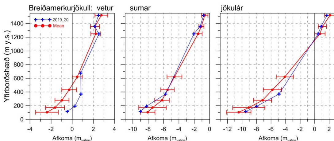
2. mynd. Breytileiki afkomu með hæð á Breiðamerkurjökli jökulárið 2019-20 og meðaltal allra ára sem afkoma hefur verið mæld (flestar ár frá 1995-96, afkoma í m vatns og hæð mælistaða í m yfir sjó). Þverstrikin sýna staðalfrávik mæliraðar í mælistöðvunum.
