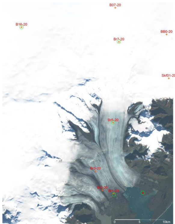
1. mynd. Afkomumælistaðir (+), veðurstöðvar (O), GPS stöðvar (Δ) og myndavél (Δ) á og við Breiðamerkurjökul. Ísaskil Breiðamerkurjökuls sýnd með blárrí línu. (í bakgrunni er Landsat8 gervihnattamynd frá 1. október 2020).
