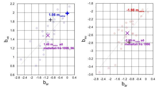
5. mynd. Ársafkoma ( b_{ár} ) Breiðamerkurjökuls teiknuð á móti vetrarafkomu ( b_{ve} , vinstri) og sumarafkomu ( b_{su} , hægri). Mæligildi jökulársins 2019_20 eru merkt með svörtum +.
